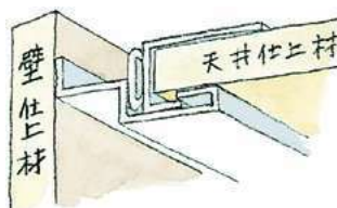
壁と天井が寄った場合 (軟質部分がつぶれた状態)
