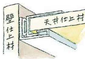
壁と天井が寄った場合 (軟質部分がつぶれた状態)
