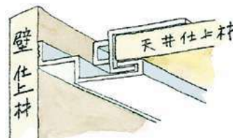
壁と天井が離れた場合 (軟質部分が離れた状態)
