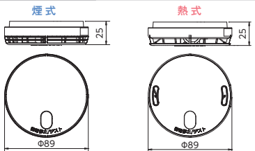
寸法図(単位mm)
