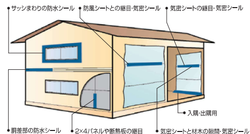
サッシまわりの防水シール (エースクロス011黒使用)
