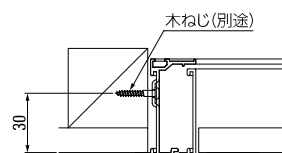
木下地納まり図
