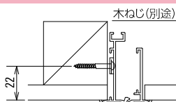
木下地納まり図
