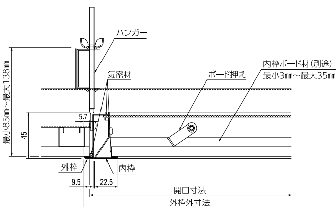
納まり図
