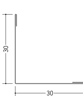
63189 L-30 (内ハゼ) 1.82m/アエンメッキ銅板 t=0.27mm
