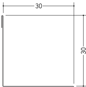
63188 L-30 (外ハゼ) 1.82m/アエンメッキ銅板 t=0.27mm
