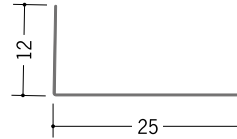
63209 L-1225 1.82m/アエンメッキ銅板 t=0.27mm
