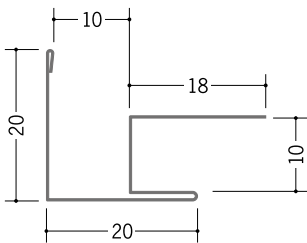
63153 亜鉛出隅 9A 1.82m/アエンメッキ銅板 t=0.27mm
