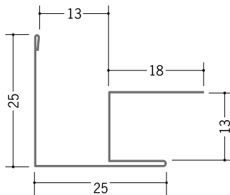
63154 亜鉛出隅 12A 1.82m/アエンメッキ銅板 t=0.27mm
