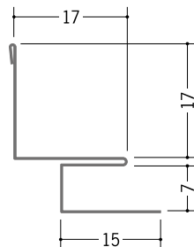
63157 亜鉛入隅 6B 1.82m/アエンメッキ銅板 t=0.27mm
