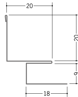
63158 亜鉛入隅 8B 1.82m/アエンメッキ銅板 t=0.27mm
