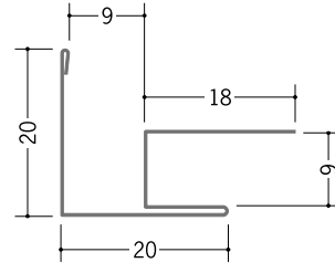
63152 亜鉛出隅 8A 1.82m/アエンメッキ銅板 t=0.27mm
