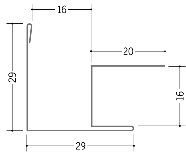
63155 亜鉛出隅 15A 1.82m/アエンメッキ銅板 t=0.27mm
