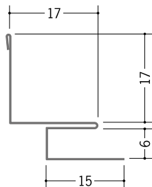
63156 亜鉛入隅 5B 1.82m/アエンメッキ銅板 t=0.27mm
