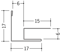
63150 亜鉛出隅 5A 1.82m/アエンメッキ銅板 t=0.27mm
