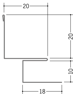
63159 亜鉛入隅 9B 1.82m/アエンメッキ銅板 t=0.27mm
