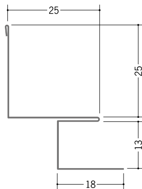
63160 亜鉛入隅 12B 1.82m/アエンメッキ銅板 t=0.27mm
