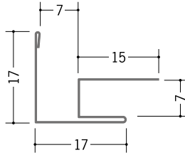
63151 亜鉛出隅 6A 1.82m/アエンメッキ銅板 t=0.27mm
