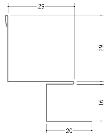
63161 亜鉛入隅 15B 1.82m/アエンメッキ銅板 t=0.27mm
