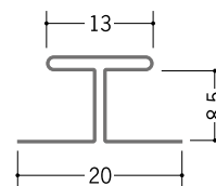
63213 H-8.5 1.82m / アエンメッキ銅板 t=0.27 mm
