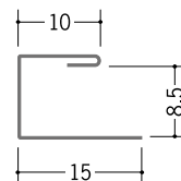
63203 コ型ハゼ付 8.5 1.82m / アエンメッキ銅板 t=0.27 mm
