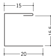
63206 コ型ハゼ付 15.5 1.82m / アエンメッキ銅板 t=0.27 mm
