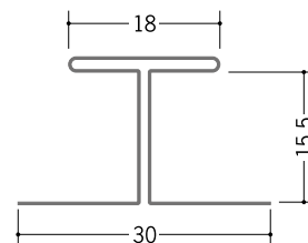
63216 H-15.5 1.82m / アエンメッキ銅板 t=0.27 mm
