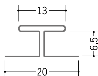
63212 H-6.5 1.82m / アエンメッキ銅板 t=0.27 mm
