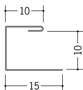
63204 コ型ハゼ付 10 1.82m / アエンメッキ銅板 t=0.27 mm
