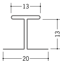
63215 H-13 1.82m / アエンメッキ銅板 t=0.27 mm
