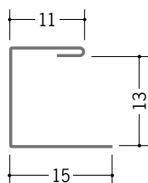
63205 コ型ハゼ付 13 1.82m / アエンメッキ銅板 t=0.27 mm
