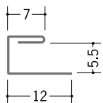
63201 コ型ハゼ付 5.5 1.82m / アエンメッキ銅板 t=0.27 mm
