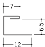
63202 コ型ハゼ付 6.5 1.82m / アエンメッキ銅板 t=0.27 mm
