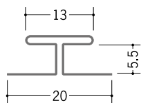
63211 H-5.5 1.82m / アエンメッキ銅板 t=0.27 mm
