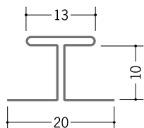
63214 H-10 1.82m / アエンメッキ銅板 t=0.27 mm
