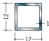
20056 ステン角パイプ 12×12 2m/ヘアライン
