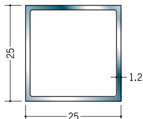
20059 ステン角パイプ 25×25 2.5m/ヘアライン
