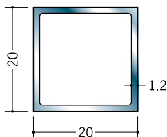
20058 ステン角パイプ 20×20 2.5m/ヘアライン
