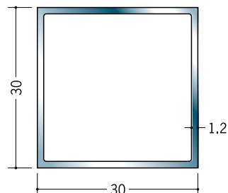
20205 ステン角パイプ 30×30 2.5m/ヘアライン
