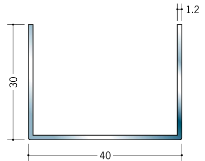
20178 ステンチャンネル 1.2×30×40 3m/ヘアライン
