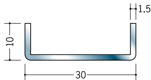
20026 ステンチャンネル 1.5×10×30 3m/ヘアライン
