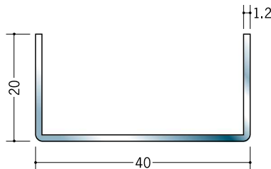
20027 ステンチャンネル 1.2×20×40 3m/ヘアライン
