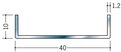
20123 ステンチャンネル 1.2×10×40 3m/ヘアライン
