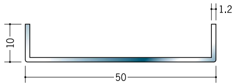
20124 ステンチャンネル 1.2×10×50 3m/ヘアライン
