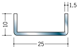
20025 ステンチャンネル 1.5×10×25 3m/ヘアライン
