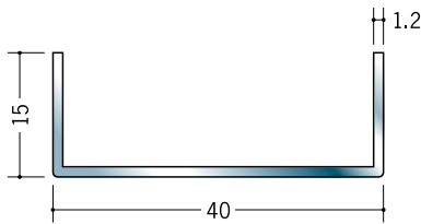
20177 ステンチャンネル 1.2×15×40 3m/ヘアライン
