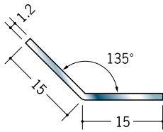
20195 ステンアングル 15-135° 3m/ヘアライン
