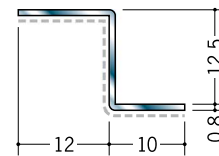
63127 ステンZバー S-1212 3m/ヘアライン
