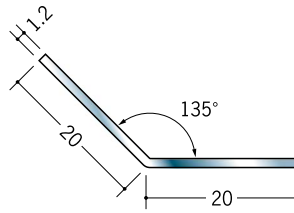
20196 ステンアングル 20-135° 3m/ヘアライン
