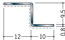
63126 ステンZバー S-912 3m/ヘアライン
