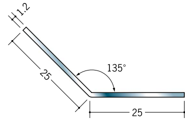
20197 ステンアングル 25-135° 3m/ヘアライン
