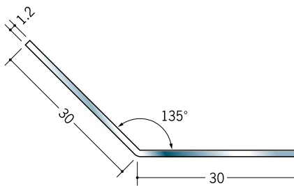
20198 ステンアングル 30-135° 3m/ヘアライン
