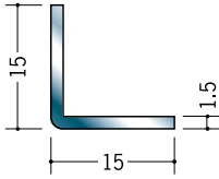
20039 ステンアングル 1.5×15×15 3m/ヘアライン
