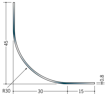
20069 ステンアングル SL45-30R 3m/ヘアライン
