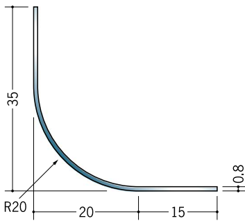
20067 ステンアングル SL35-20R 3m/ヘアライン
