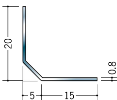
20015 ステン5mm面取 アングル 20 3m/ヘアライン
