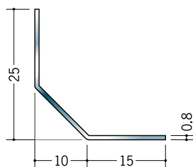
20016 ステン10mm面取 アングル 25 3m/ヘアライン
