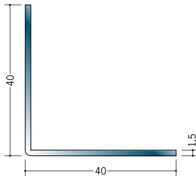
20038 ステンアングル 1.5×40×40 3m/ヘアライン
