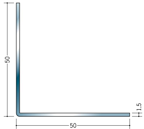
20048 ステンアングル 1.5×50×50 3m/ヘアライン
