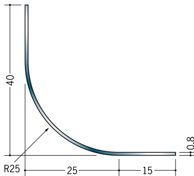
20068 ステンアングル SL40-25R 3m/ヘアライン
