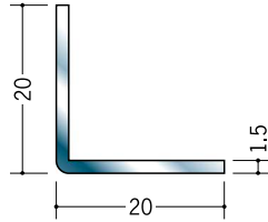
20035 ステンアングル 1.5×20×20 3m/ヘアライン
