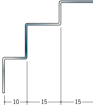
64052 ステン角型入隅9.5 2.73m / ヘアーライン・鏡面 (#800) t=0.8mm
