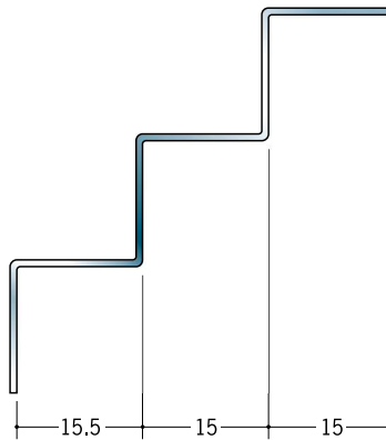
64054 ステン角型入隅16 2.73m / ヘアーライン・鏡面 (#800) t=0.8mm
