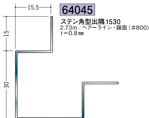
上段 鏡面 (#800) 下段 ヘアライン
