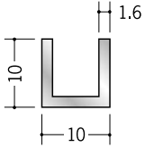
58089 アルミチャンネル 1.6×10×10 2m/アルマイトシルバー
