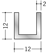
58264 アルミチャンネル 2×12×12 2m (−3 mm, +5 mm) アルマイトシルバー
