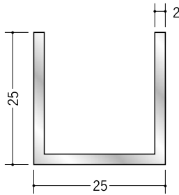
58084 アルミチャンネル 2×25×25 2m/アルマイトシルバー
