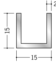
58088 アルミチャンネル 2×15×15 2m/アルマイトシルバー
