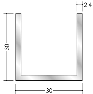
56346 アルミチャンネル 2.4×30×30 2m/アルマイトシルバー
