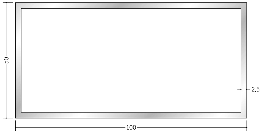
56338 アルミ角パイプ 2.5×50×100 2.5m／アルマイトシルバー
