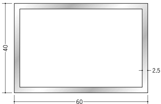
56337 アルミ角パイプ 2.5×40×60 2.5m (−3 mm, +5 mm) アルマイトシルバー
