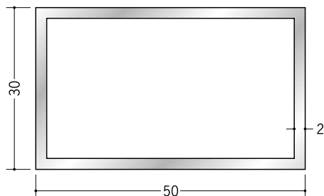
56333 アルミ角パイプ 2×30×50 2.5m (−3 mm, +5 mm) アルマイトシルバー
