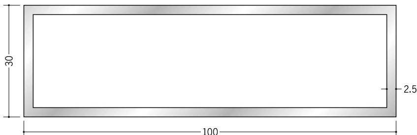
56336 アルミ角パイプ 2.5×30×100 2.5m (−3 mm, +5 mm) アルマイトシルバー
