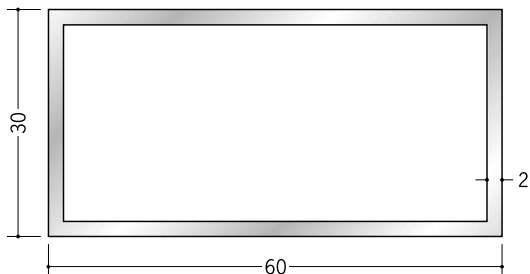
56334 アルミ角パイプ 2×30×60 2.5m (−3 mm, +5 mm) アルマイトシルバー
