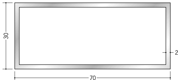
56335 アルミ角パイプ 2×30×70 2.5m (−3 mm, +5 mm) アルマイトシルバー
