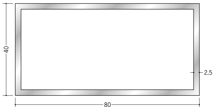
58072 アルミ角パイプ 2.5×40×80 2.5m (−3 mm, +5 mm) アルマイトシルバー
