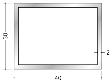
56332 アルミ角パイプ 2×30×40 2.5m (−3 mm, +5 mm) アルマイトシルバー
