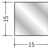
58048 アルミ角棒 15×15 2m (−3mm, +5mm) アルマイトシルバー
