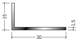
28053 アルミカラーアングル 1.5×15×30BW 3m／ホワイトアルマイト1 電解ブラック
