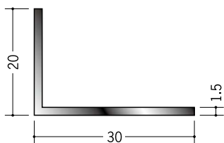
28055 アルミカラーアングル 1.5×20×30BW 3m／ホワイトアルマイト1 電解ブラック
