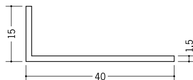
28056 アルミカラーアングル 1.5×15×40BW 3m／ホワイトアルマイト1 電解ブラック
