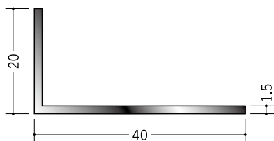
28054 アルミカラーアングル 1.5×20×40BW 3m／ホワイトアルマイト1 電解ブラック
