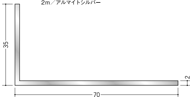
56276 アルミアングル 2×35×70 2m/アルマイトシルバー
