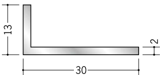
56266 アルミアングル 2×13×30 2m/アルマイトシルバー
