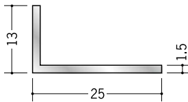
56265 アルミアングル 1.5×13×25 2m/アルマイトシルバー
