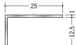
56161 アルミアングル 1×13.5×25 2m/アルマイトシルバー
