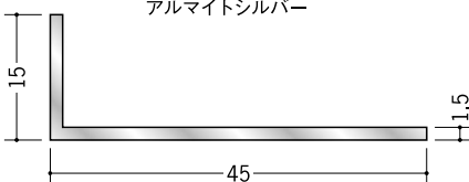
56173 アルミアングル 1.5×15×45 2m(-3mm, +5mm) アルマイトシルバー
