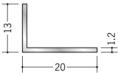
56264 アルミアングル 1.2×13×20 2m/アルマイトシルバー
