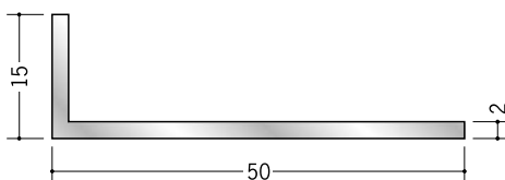
56269 アルミアングル 2×15×50 2m/アルマイトシルバー
