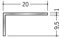
56159 アルミアングル 1×10.5×20 2m/アルマイトシルバー
