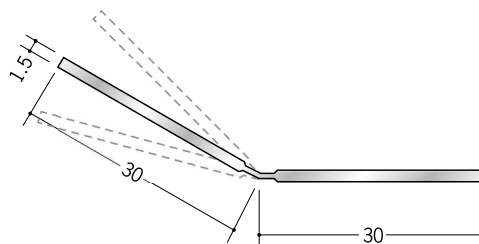
56071 アルミフリーアングル 30 2m/アルマイトシルバー
