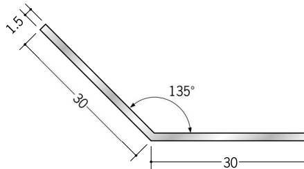
56104 アルミ角度付アングル 30 3m/アルマイトシルバー
