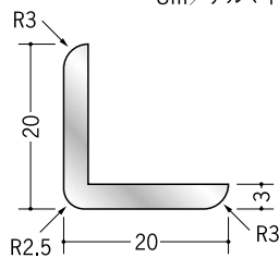
56191 アルミ出隅 アングル20-2.5R 3m/アルマイトシルバー
