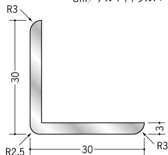
56193 アルミ出隅 アングル30-2.5R 3m/アルマイトシルバー
