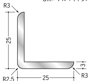
56192 アルミ出隅 アングル25-2.5R 3m/アルマイトシルバー
