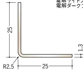
28016 アルミカラーアングル L2R25×25BR
