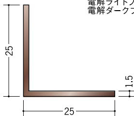
28021 アルミカラーアングル 1.5×25×25BR
