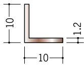
28017 アルミカラーアングル 1.2×10×10BR
