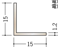
28019 アルミカラーアングル 1.2×15×15BR
