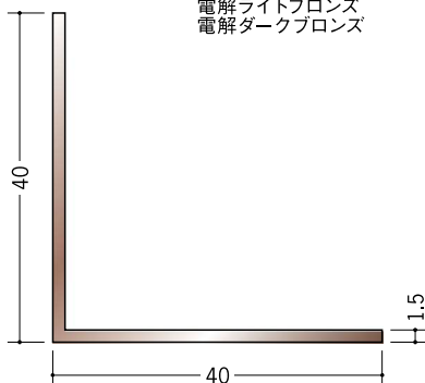
28030 アルミカラーアングル 1.5×40×40BR
