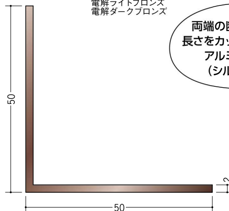
28023 アルミカラーアングル 2×50×50BR
