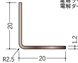
28015 アルミカラーアングル L2R20×20BR
