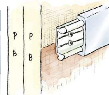
79142 アルミモール KW-40 用キャップ ビニール／t=1.5mm シルバーメタリック・オフホワイト・アイボリー・コスモブラック・うす茶
