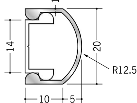
55141 腰かべモール RA-20S 2m／アルマイトシルバー ベース：ビニール
