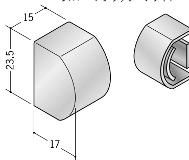
57182 腰かべモール RA-20S 用 キャップ ビニール／t=1.5mm シルバーメタリック・ホワイト・ベージュ
