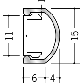
55140 腰かべモール RA-15S 2m／アルマイトシルバー ベース：ビニール
