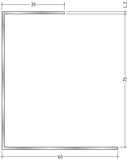
51036 アルミ A 型 75 3m / アルマイトシルバー
