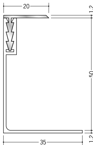
35084 CF-2 (コ型ベース 50mm 用) 1.82m / ホワイト / 50 本入
