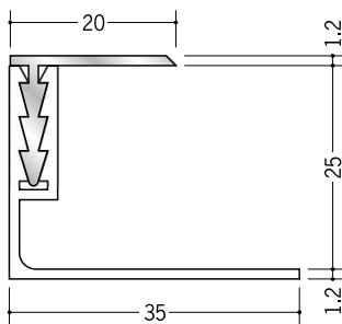
35083 CF-1 (コ型ベース 25mm 用) 1.82m / ホワイト / 50 本入
