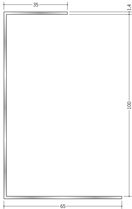
51181 アルミ A 型 100 3m / アルマイトシルバー
