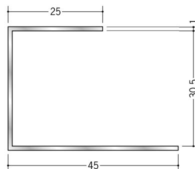
51037 アルミ A型 30 3m/アルマイトシルバー
