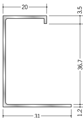
51028 アルミ A型 36 3m/アルマイトシルバー
