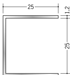
54265 アルミ コ型 25BS 3m/アルマイトシルバー
