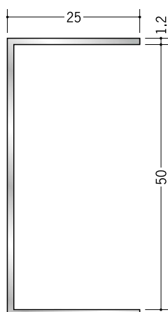
54268 アルミ コ型 50BS 3m/アルマイトシルバー
