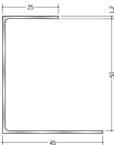
51038 アルミ A型 50 3m/アルマイトシルバー
