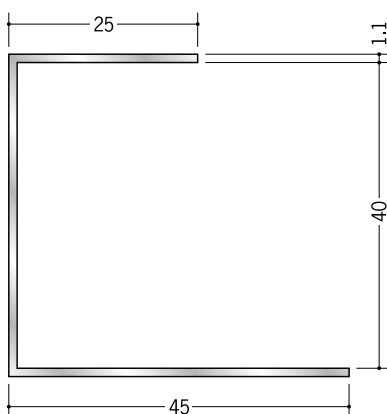
51035 アルミ A型 40 3m/アルマイトシルバー
