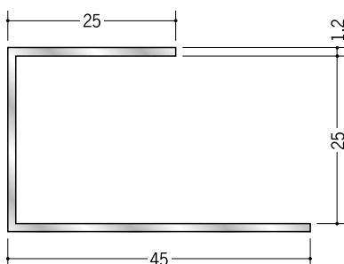
51034 アルミ A型 25 3m/アルマイトシルバー
