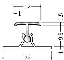
55064 カンゴウAKT-9.5 2.73m / アルマイトシルバー ベース：ビニール
