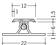
52160 カンゴウAKT-6.5 2.73m / アルマイトシルバー ベース：ビニール
