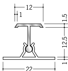
55065 カンゴウAKT-12.5 2.73m / アルマイトシルバー ベース：ビニール
