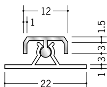
58234 カンゴウAKT-3.5 2.73m / アルマイトシルバー ベース：ビニール
