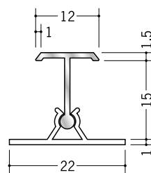
58061 カンゴウAKT-15.5 2.73m / アルマイトシルバー ベース：ビニール
