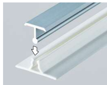
53237 カンゴウKNC-5 2.73m / アルマイトシルバー ベース：ビニール
