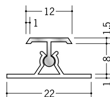
52161 カンゴウAKT-8.5 2.73m / アルマイトシルバー ベース：ビニール
