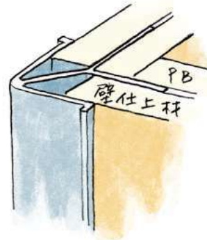
54149 アルミ F型出隅 9 3m/アルマイトシルバー
