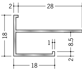
54147 アルミ F型出隅 8 3m/アルマイトシルバー
