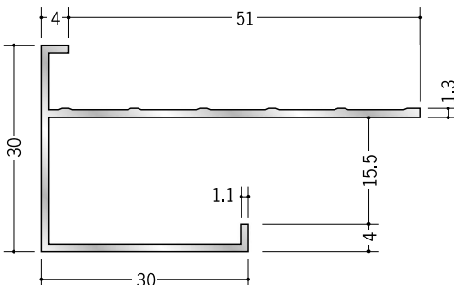
59089 アルミ F型出隅 15 3m/アルマイトシルバー
