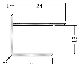
50078 アルミ 12AD 2.73m/アルマイトシルバー 3m/アルマイトシルバー
