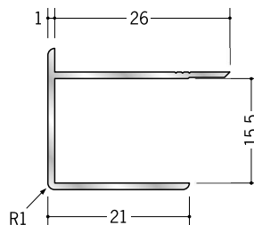
50079 アルミ 15AD 2.73m/アルマイトシルバー
