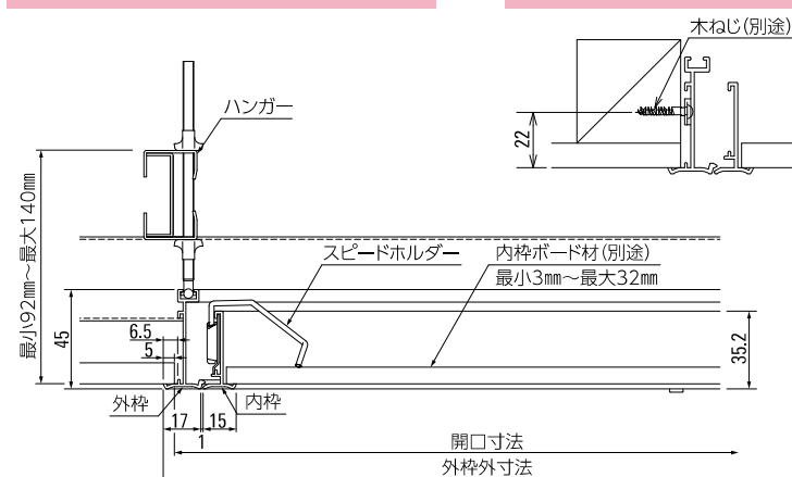
納まり図
