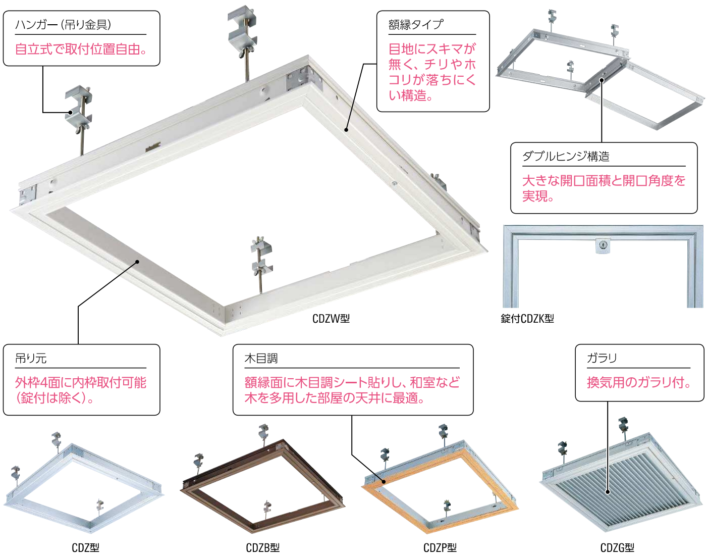
部材仕様
