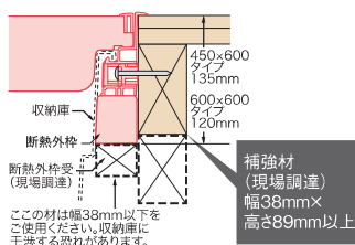
参考納まり図
