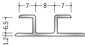
53068 アルミハット型6 2.5m/アルマイトシルバー
