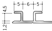
53064 アルミハット型4 2.5m/アルマイトシルバー
