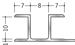
53074 アルミハット型9.5 2.5m/アルマイトシルバー
