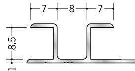
53070 アルミハット型8.5 2.5m/アルマイトシルバー
