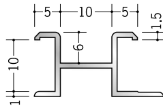
53186 アルミハット90MC 2.73m/アルマイトシルバー
