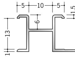
53187 アルミハット120MC 2.73m/アルマイトシルバー
