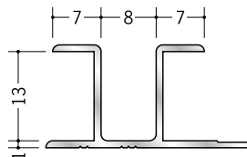
53071 アルミハット型13 2.5m/アルマイトシルバー
