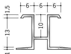
53075 アルミハット型12.5 2.5m/アルマイトシルバー
