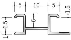
53184 アルミハット60MC 2.73m/アルマイトシルバー
