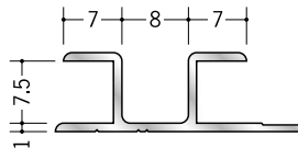
53069 アルミハット型7 2.5m/アルマイトシルバー
