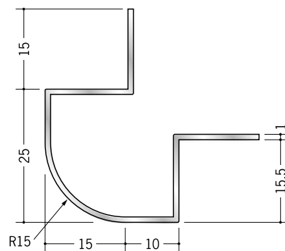
50119 アルミタコ出隅15R-15 2.73m/アルマイトシルバー
