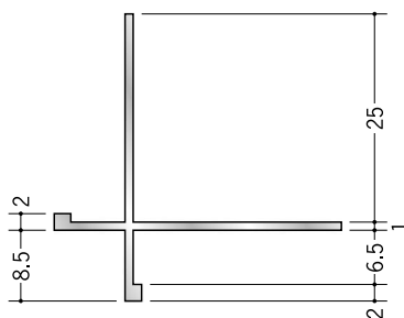
53151 アルミ XA-15.5+2 2.73m/アルマイトシルバー
