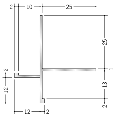
53256 アルミ XTN-1013 2.73m/アルマイトシルバー
