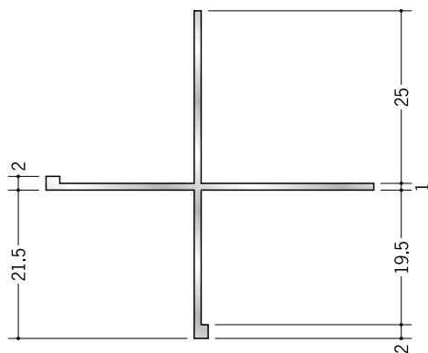
53256 アルミ XTN-1013 2.73m/アルマイトシルバー
