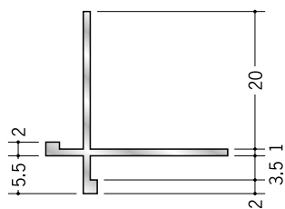
53162 アルミ XA-3.5+2 2.73m/アルマイトシルバー
