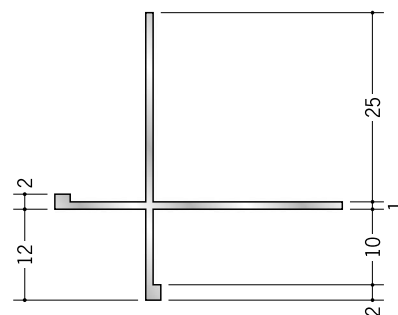
53169 アルミ XA-10+2 2.73m/アルマイトシルバー
