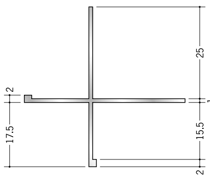
53151 アルミ XA-15.5+2 2.73m/アルマイトシルバー
