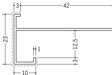
29153 アルミD型32.5 (岩綿板用) AP カラー 3m/バニラホワイト
