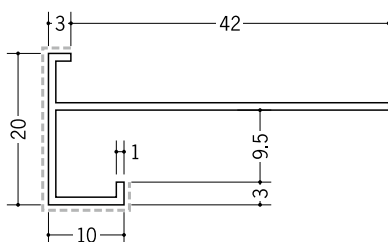
29152 アルミD型31.5 (岩綿板用) AP カラー 3m/バニラホワイト
