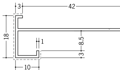
29151 アルミD型33AP カラー 3m/バニラホワイト
