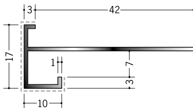
29148 アルミD型30AP カラー 3m/バニラホワイト カスタムブラック
