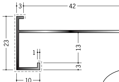
29150 アルミD型32AP カラー 3m/バニラホワイト カスタムブラック
