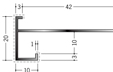
29149 アルミD型31AP カラー 3m/バニラホワイト カスタムブラック
