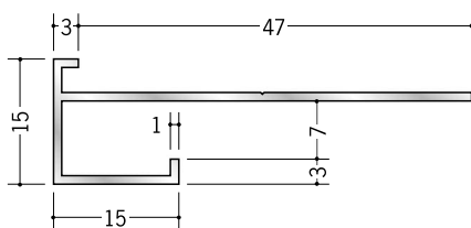
52037 アルミ D 型 37 3m / アルマイトシルバー
