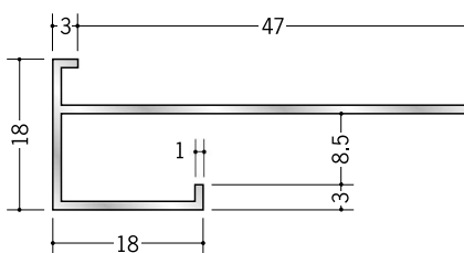
52039 アルミ D 型 39 3m / アルマイトシルバー
