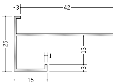
52209 アルミ D 型 78 3m / アルマイトシルバー
