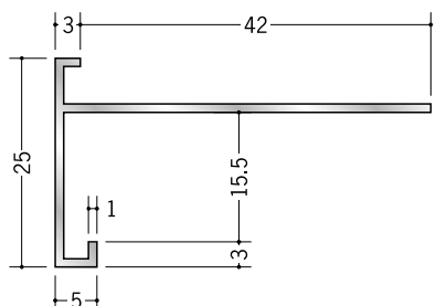
52119 アルミD型85 3m/アルマイトシルバー
