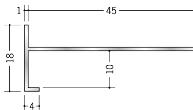
52341 アルミD型93 3m/アルマイトシルバー
