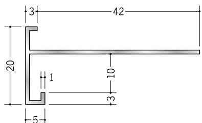
52117 アルミD型83 3m/アルマイトシルバー
