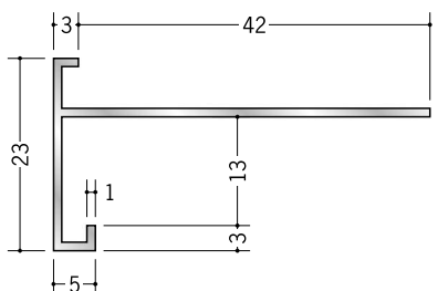
52118 アルミD型84 3m/アルマイトシルバー
