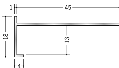
52342 アルミD型94 3m/アルマイトシルバー
