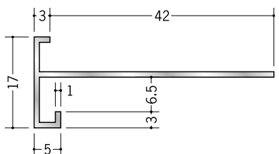
52115 アルミD型81 3m/アルマイトシルバー
