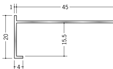
52343 アルミD型95 3m/アルマイトシルバー
