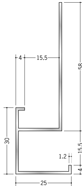
52095 アルミD型25 3m／アルマイトシルバー
