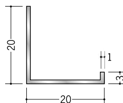
52135 アルミC型-20 3m アルマイトシルバー
