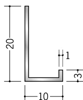
52133 アルミC型-10 3m アルマイトシルバー
