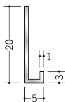
52132 アルミC型-5 3m アルマイトシルバー
