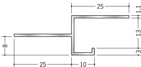
51243 アルミ換気見切 KML-13 3m/アルマイトシルバー 開口率 22.03%
