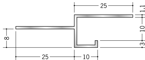
51242 アルミ換気見切 KML-10 3m/アルマイトシルバー 開口率 22.03%
