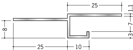
51241 アルミ換気見切 KML-7 3m/アルマイトシルバー 開口率 22.03%
