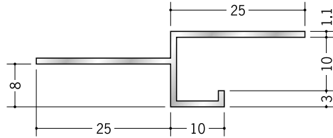
51237 アルミ換気見切 KMO-10 3m/アルマイトシルバー 開口率 15.07%
