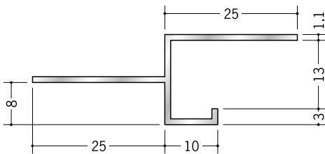
51238 アルミ換気見切 KMO-13 3m/アルマイトシルバー 開口率 15.07%
