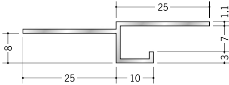
51236 アルミ換気見切 KMO-7 3m/アルマイトシルバー 開口率 15.07%
