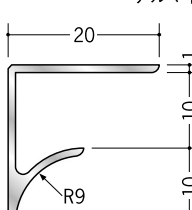
54516 アルミ NR-10 2.73m アルマイトシルバー
