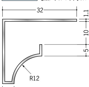
52024 アルミ RSB-9.5 3m / アルマイトシルバー
