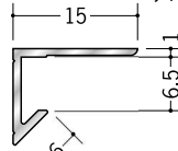
55005 アルミ型 6.5 2.73m アルマイトシルバー
