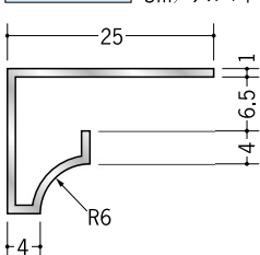
52001 アルミ RSA-6 3m / アルマイトシルバー
