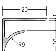
54512 アルミ NR-4.5 2.73m アルマイトシルバー
