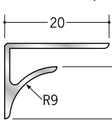
54511 アルミ NR-3.5 2.73m アルマイトシルバー
