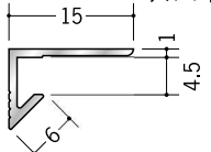
55003 アルミ型 4.5 2.73m アルマイトシルバー
