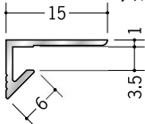
55002 アルミ型 3.5 2.73m アルマイトシルバー
