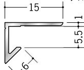
55004 アルミ型 5.5 2.73m アルマイトシルバー
