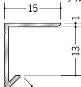
55008 アルミ型 13 2.73m アルマイトシルバー
