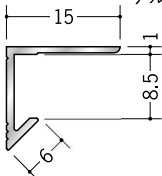
55006 アルミ型 8.5 2.73m アルマイトシルバー
