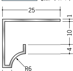
52003 アルミ RSA-9 3m / アルマイトシルバー
