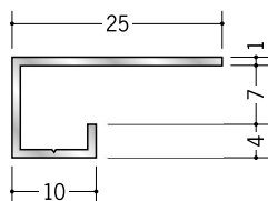
51004 アルミ A 型7 (中) 3m/アルマイトシルバー
