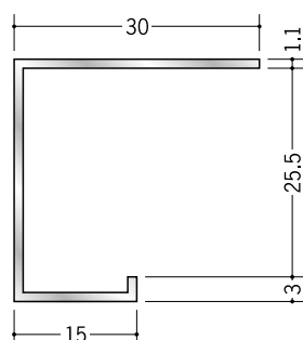
51140 アルミ A 型25.5 3m/アルマイトシルバー
