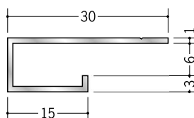
15 51030 アルミ A 型6 (大) 3m/アルマイトシルバー
