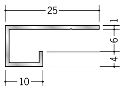
10 51014 アルミ A 型6 3m/アルマイトシルバー
