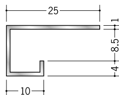
51018 アルミ A 型13 (小) 3m/アルマイトシルバー
