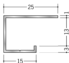
51140 アルミ A 型25.5 3m/アルマイトシルバー
