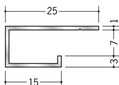
51031 アルミ A 型9.5 (大) 3m/アルマイトシルバー
