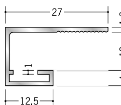
51094 アルミ SA-10 3m/アルマイトシルバー
