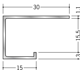
51025 アルミ A 型15 3m/アルマイトシルバー
