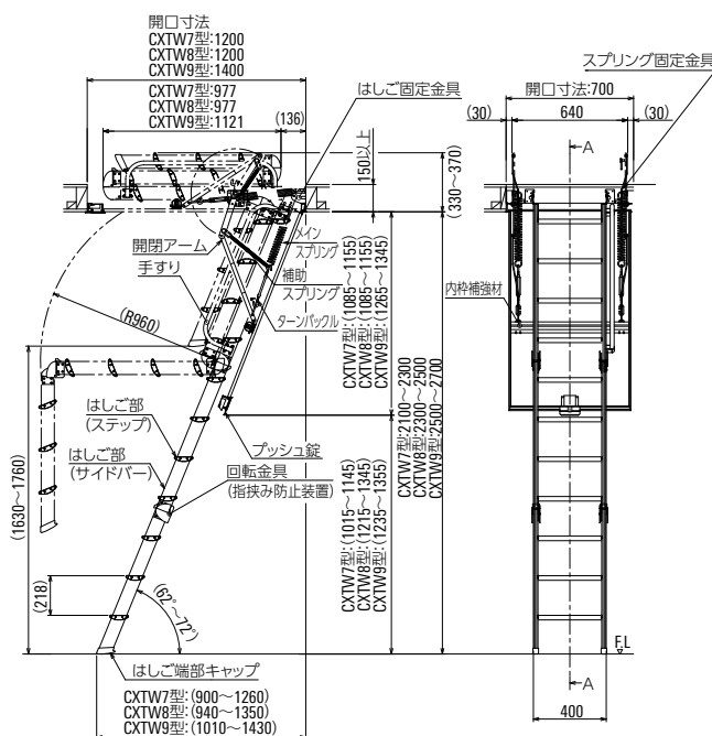
■AA断面
