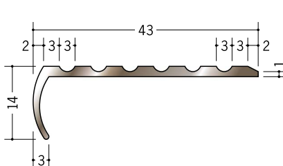
61607 アルミノンスリップA43DB 2.73m/電解ダークブロンズ
