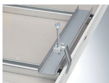
①ハンガーを外枠にセット
