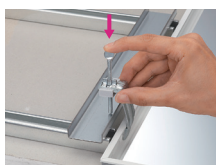
②ハンガーボルトを取付野縁に当たるところまで押し込む
