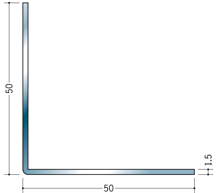
20048 ステンアングル 1.5×50×50 3m/ヘアーライン
