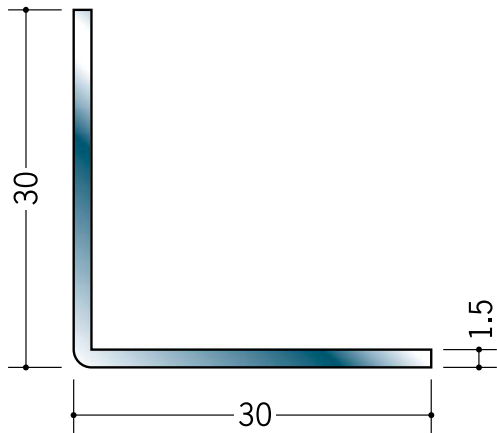
20037 ステンアングル 1.5×30×30 3m/ヘアーライン
