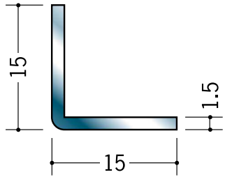
20039 ステンアングル 1.5×15×15 3m/ヘアーライン
