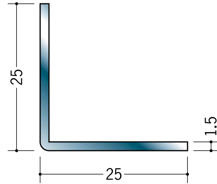
20036 ステンアングル 1.5×25×25 3m/ヘアーライン
