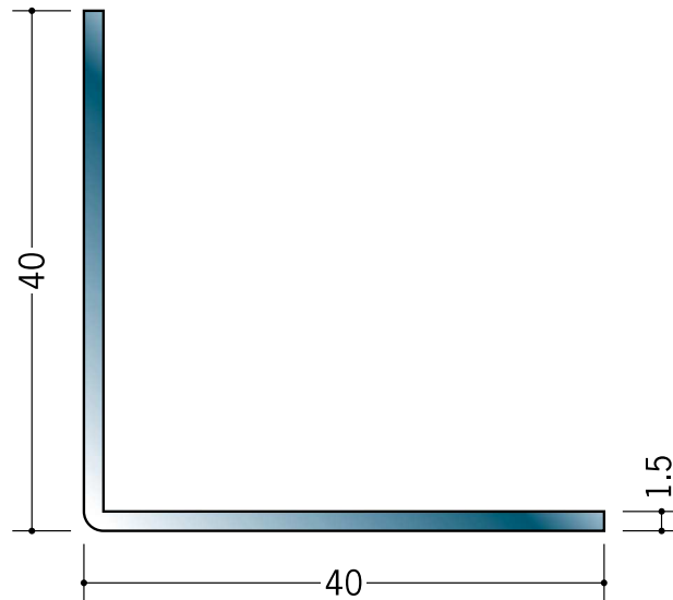
20038 ステンアングル 1.5×40×40 3m/ヘアーライン
