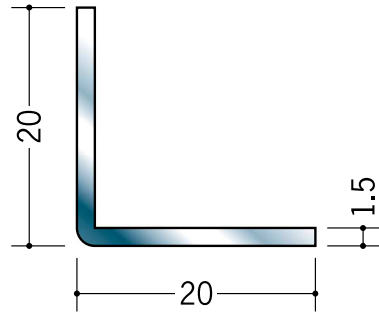
20035 ステンアングル 1.5×20×20 3m/ヘアーライン
