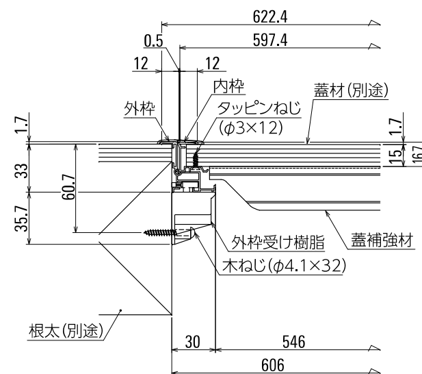
納まり図
