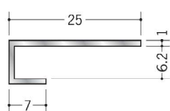
54301 アルミ ACS-6 3m/アルマイトシルバー
