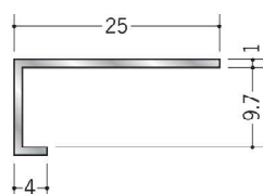
50032 アルミ ATC-10 3m/アルマイトシルバー
