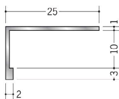
52128 アルミ LSC-10 3m/アルマイトシルバー
