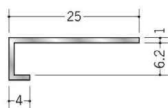
50030 アルミ ATC-7 3m/アルマイトシルバー
