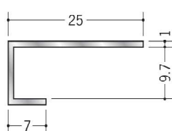
54303 アルミ ACS-9 3m/アルマイトシルバー
