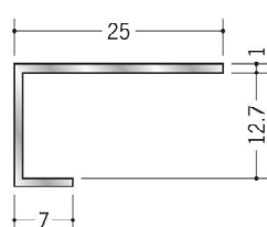
54304 アルミ ACS-12 3m/アルマイトシルバー
