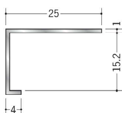
50034 アルミ ATC-15 3m/アルマイトシルバー
