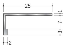
52126 アルミ LSC-7 3m/アルマイトシルバー
