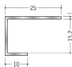
54315 アルミ ACT-15 3m/アルマイトシルバー
