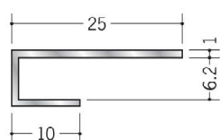
54311 アルミ ACT-6 3m/アルマイトシルバー
