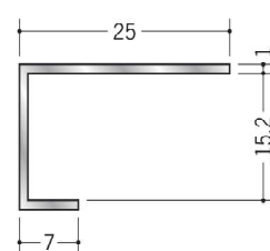
54305 アルミ ACS-15 3m/アルマイトシルバー
