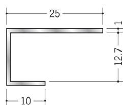
54314 アルミ ACT-12 3m/アルマイトシルバー
