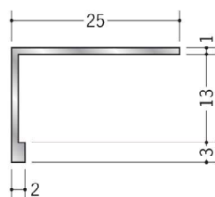
52129 アルミ LSC-13 3m/アルマイトシルバー
