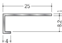
50031 アルミ ATC-8 3m/アルマイトシルバー
