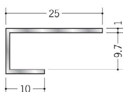
54313 アルミ ACT-9 3m/アルマイトシルバー
