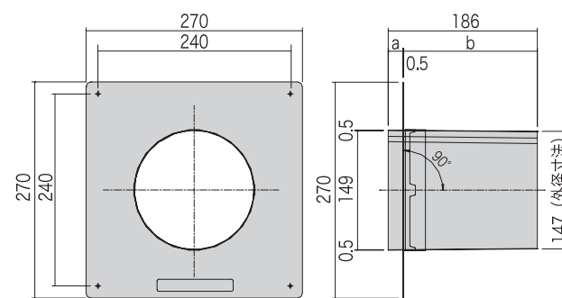
不燃パイプφ150
