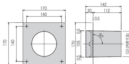
不燃パイプφ100
